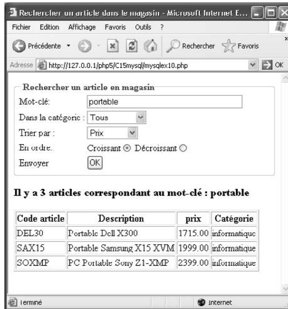
Figure 15-8 Formulaire de recherche et résultats obtenus
