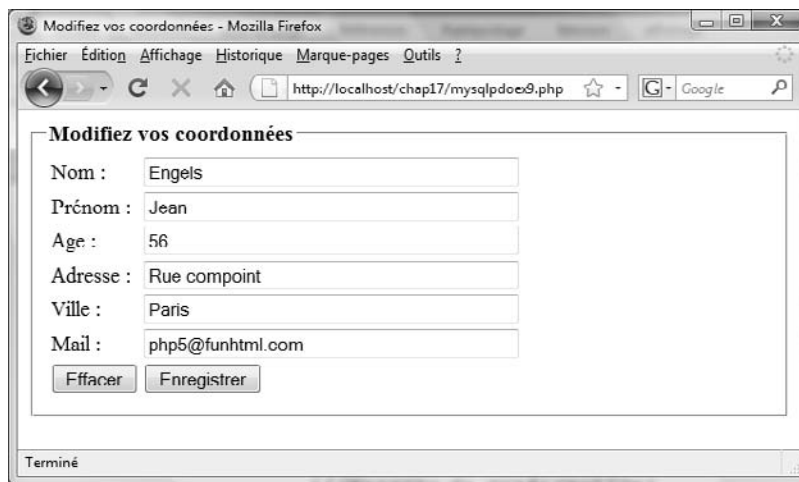
Figure 17-7 Formulaire de saisie des coordonnées créé dynamiquement
