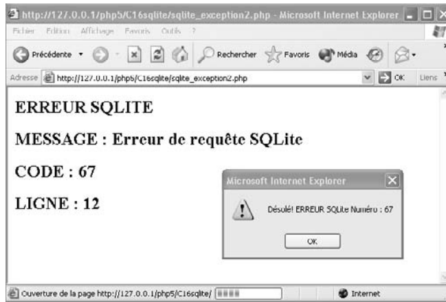
Figure 18-6 Résultat obtenu en cas d'erreur
